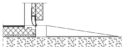
Rom uten gulv -Standard dør med slepelist -Standard maskinelement
