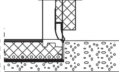
Nedsenket gulv -Forkortet dørblad med slepelist -Redusert høyde maskinelement
