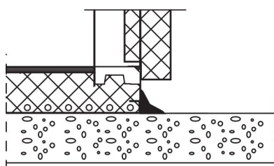
Standard gulvløsning -Standard dør -Standard maskinelement
