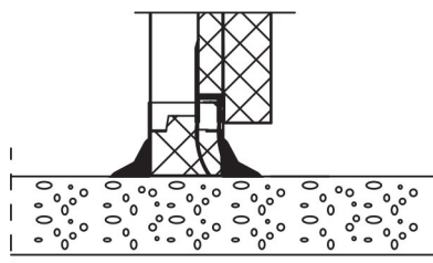
Rom uten gulv -Standard dør med slepelist -Standard maskinelement
