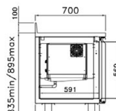
Topplate med oppkant
