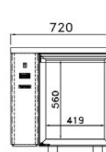
Breddemål sentralkjøl
