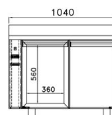
Breddemål sentralkjøl
