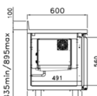
Topplate med oppkant
