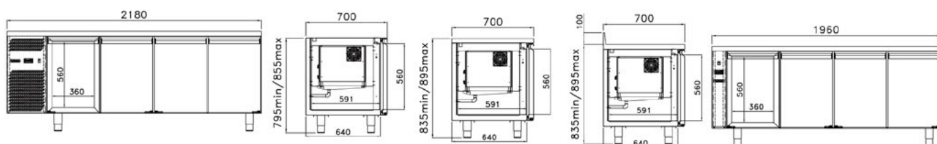
Breddemål
