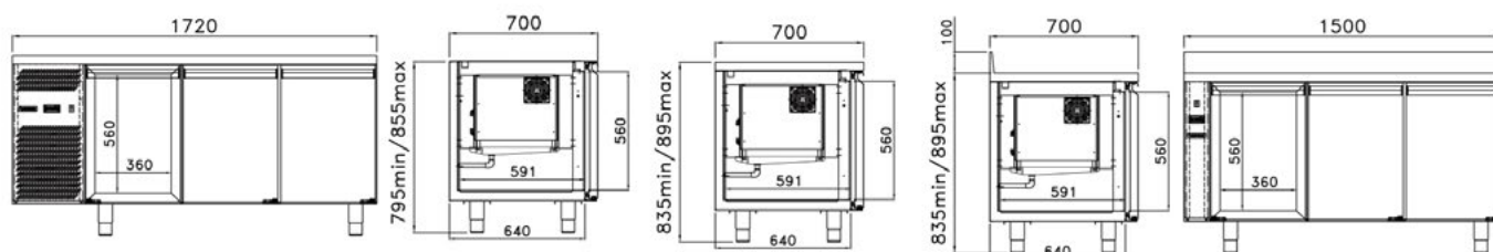
Breddemål
